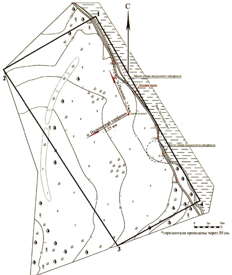
Инструментальный план стоянки Верх-Исетская VII (Правобережная).
