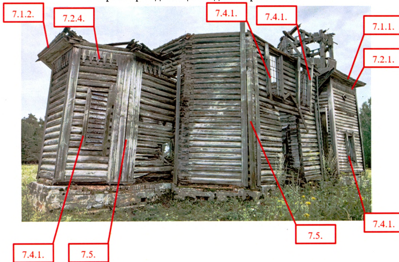
Северный фасад. Общий вид с северо-востока
