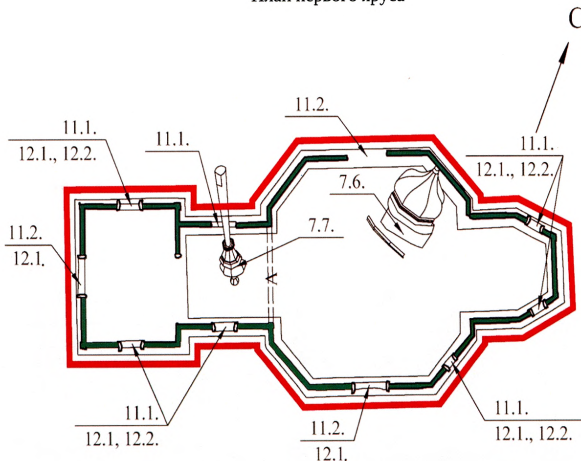
План первого яруса
