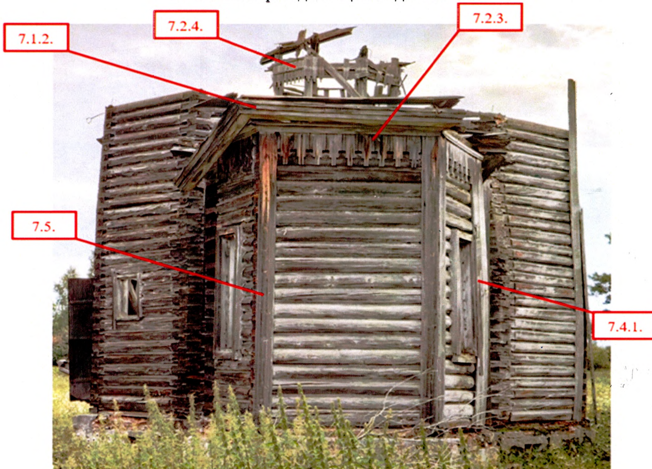
Восточный фасад. Общий вид с востока
