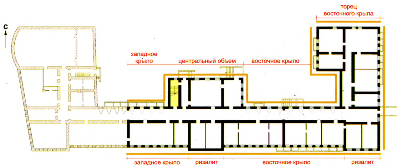
План подвала
