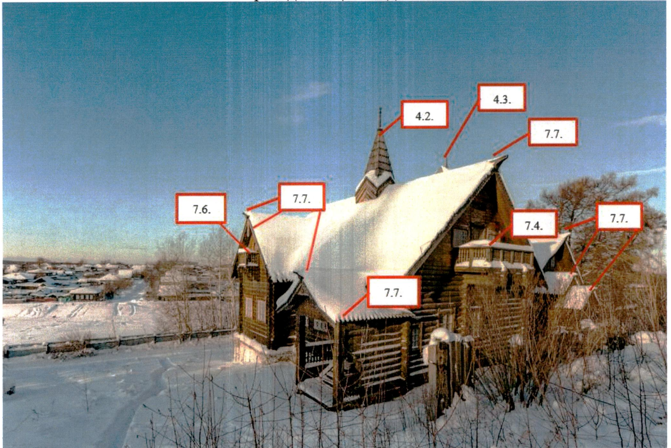
Восточный фасад. Общий вид с юго-востока
