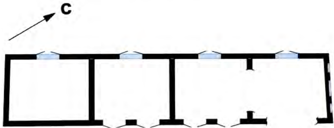
План 1 этажа
