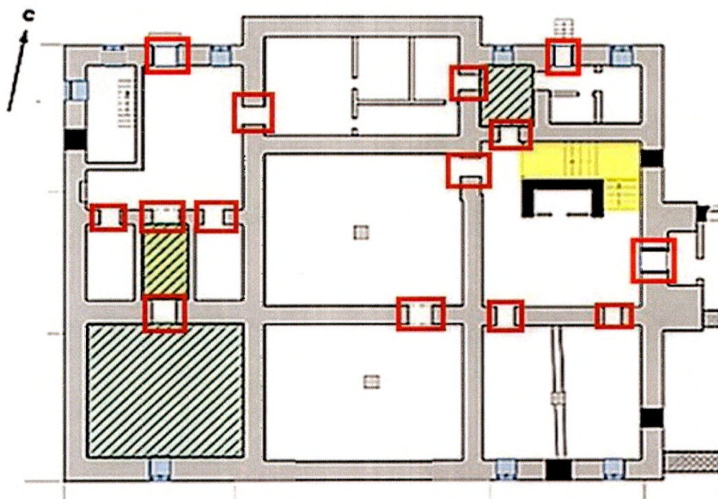
План подвала
