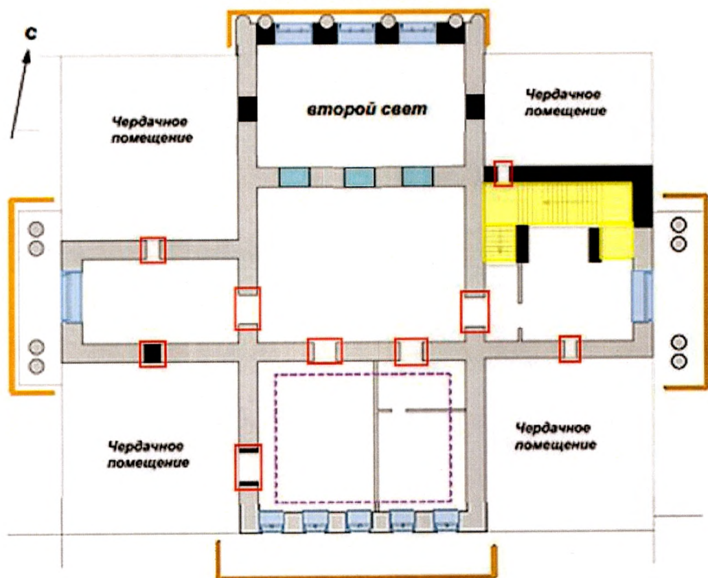
План мезонина
