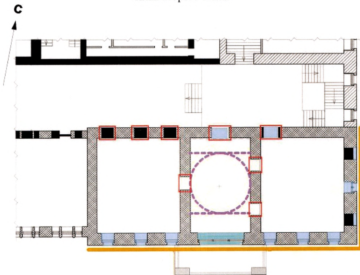
План второго этажа
