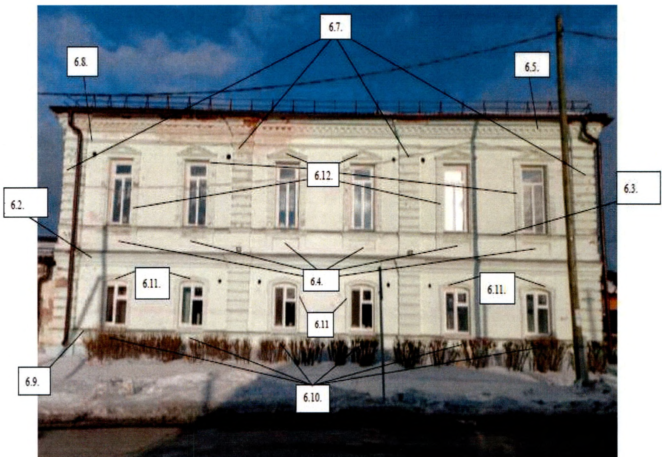
Западный фасад
